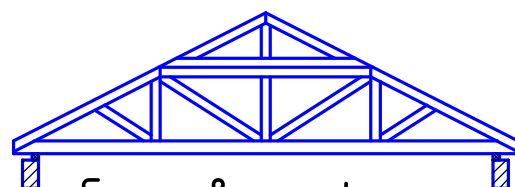
Составная ферма
