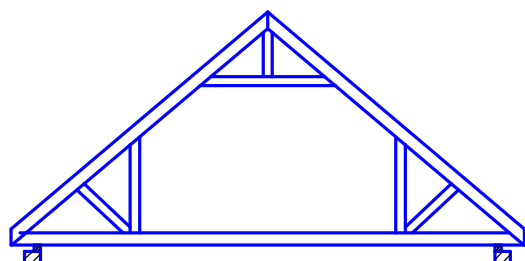
Мансардная рама
